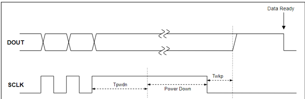
图 5: 掉电模式时序图
