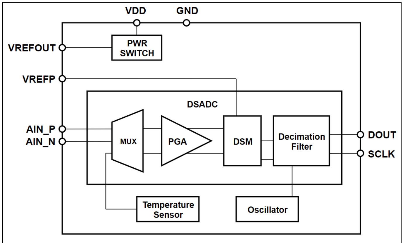
图 1: PMD040B 图框
