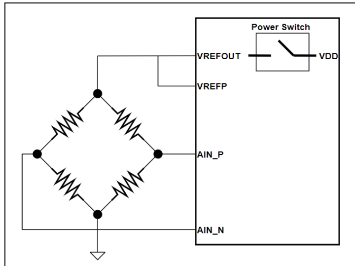
图 4: 高压侧电源开关示意图
